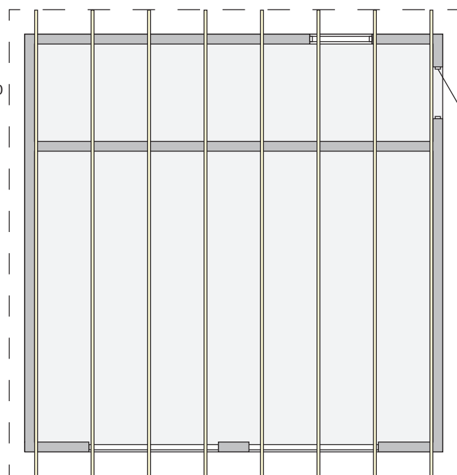
TAKBJELKEPLAN
